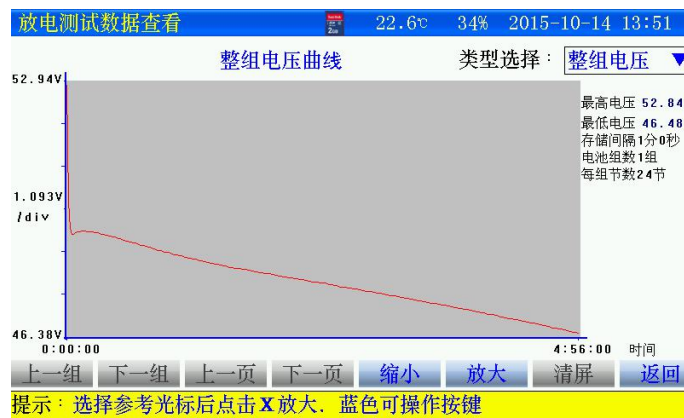
图 3.5.4 整组电压曲线界面
